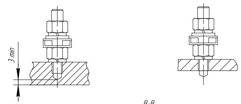
А-А (разрезано) Внутренний зажим заземления ГОСТ21130 Б-Б (разрезано) Внешний зажим заземления ГОСТ21130
