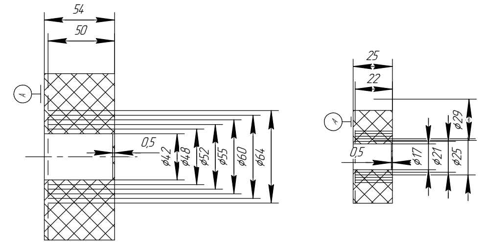
Кольцо резиновое уплотнительное кабельного ввода Резина ИРП 1054 силикон Кольцо резиновое уплотнительное дополнительного ввода Резина ИРП 1054 силикон
