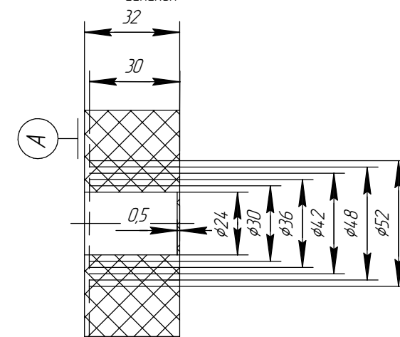
Кольцо резиновое уплотнительное кабельного ввода Резина ИРП 1054 силикон
