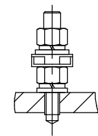
Б-Б (разрезано) Внешний зажим заземления ГОСТ21130
