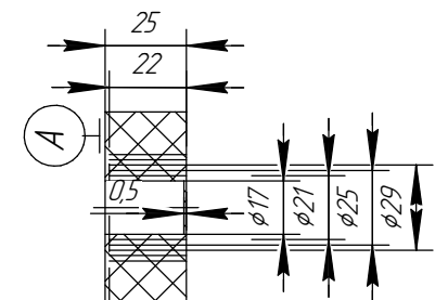
Кольцо резиновое уплотнительное сервисного кабельного ввода Резина ИРП 1054 силикон
