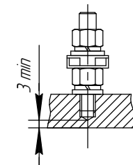
А-А (разрезано) Внутренний зажим заземления ГОСТ21130
