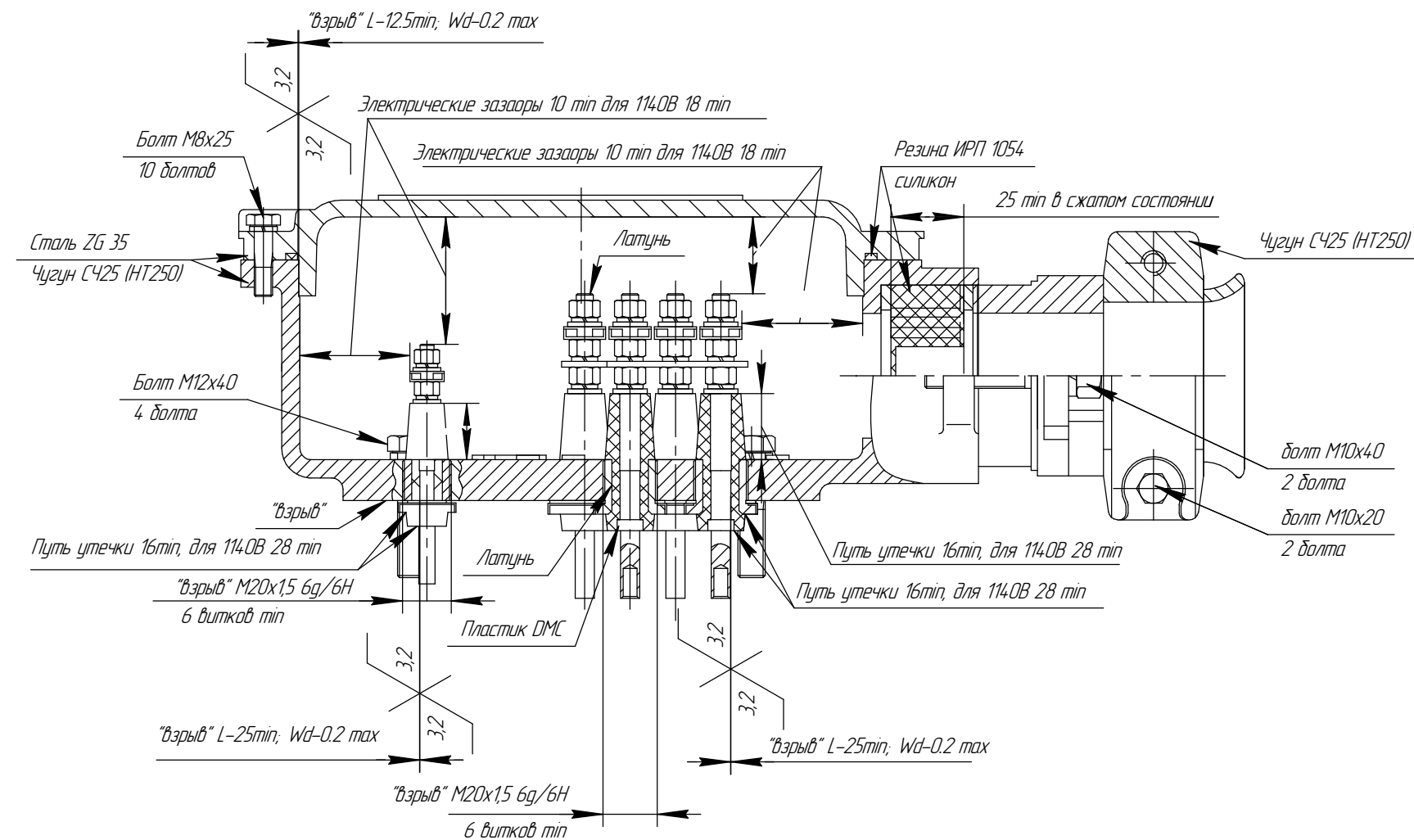
А-А (разрезано) Внутренний зажим заземления ГОСТ21130
