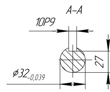
Рисунок В.4 (обязательное) Габаритные, установочные и присоединительные размеры двигателей АИМУ основного исполнения. (с удлиненным валом АИМУ 132)
