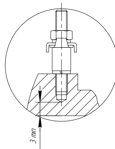
Чертеж Д.1 Вводное устройство М4 электродвигателя АИМУ 63-80
