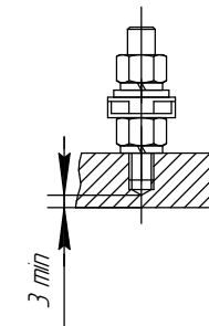
А-А внутренний заземляющий зажим ГОСТ 21130
