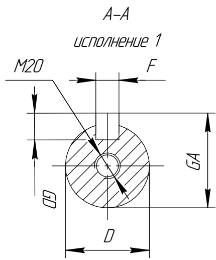
Рисунок В.9 Габаритные, установочные и присоединительные размеры двигателей АИМУ основного исполнения. Габарит 200-280. Монтажное исполнение IM 1001, IM 1011, IM 1031
