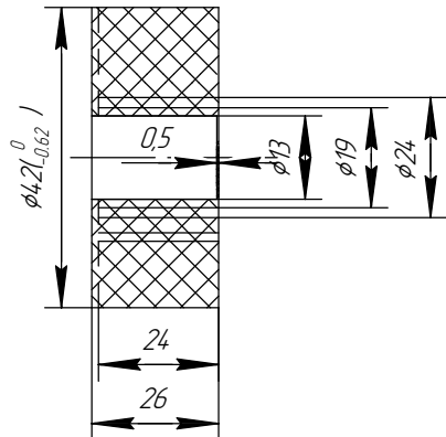
Резиновое разжимное кольцо Резина ИРП 1054 Силикон ИРП 1338
