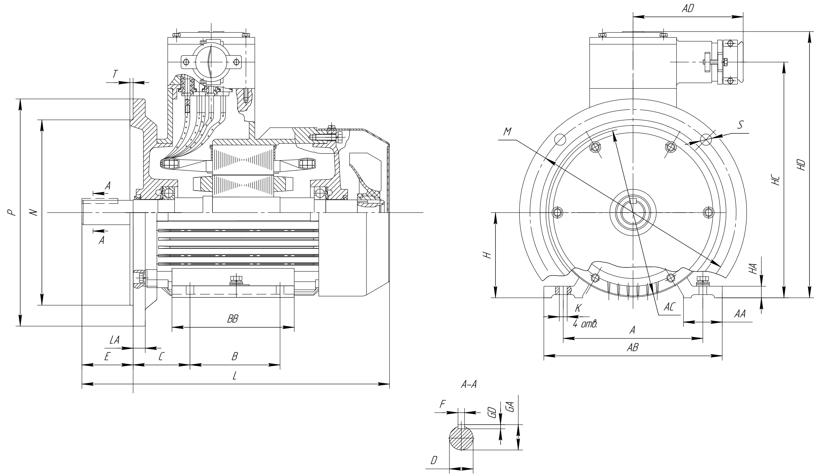
Рисунок В.2 (обязательное) Габаритные, установочные и присоединительные размеры двигателей АИМУ 63-180 основного исполнения. Монтажное исполнение IM 2001, IM 2081
