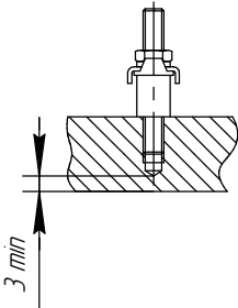
А-А внутренний заземляющий зажим ГОСТ 21130
