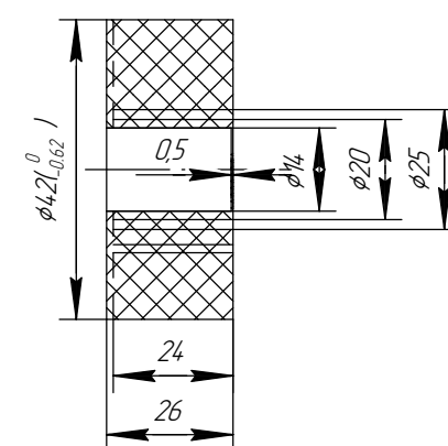
Резиновое разжимное кольцо Резина ИРП 1054 Силикон ИРП 1338
