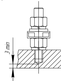
A-A Внутренний зажим заземления ГОСТ21130
