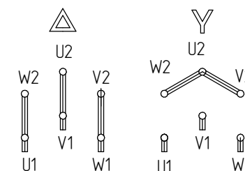
Схема подключения
