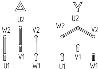
Схема подключения
