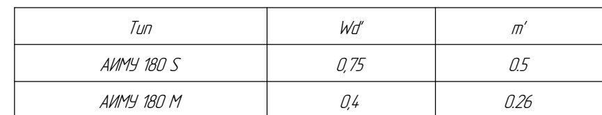
Чертеж Г.26 Электродвигатель асинхронный взрывозащищенный АИМУ 180
